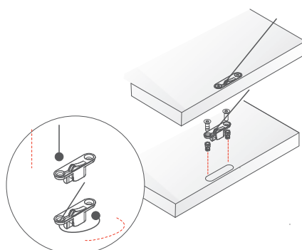
Fixação do engate embutido
