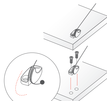
Fixação do engate saliente
