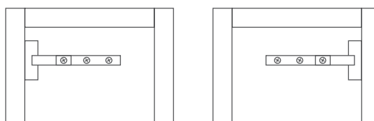
Fixação na lateral do móvel (ambidestro)
