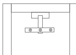
Fixação no tampo do móvel
